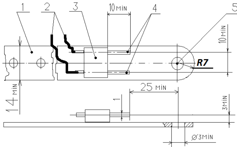
Мал. 1. Побудова кордової планки з контактами:
